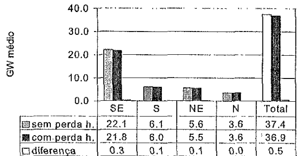
Figura 4 – Efeito das perdas hidráulicas na energia firme
