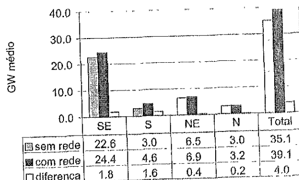
Figura 1 - Efeito das interconexões na energia firme
