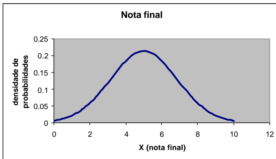
Figura 2 Densidade de probabilidade da nota final, média das 20 avaliações
